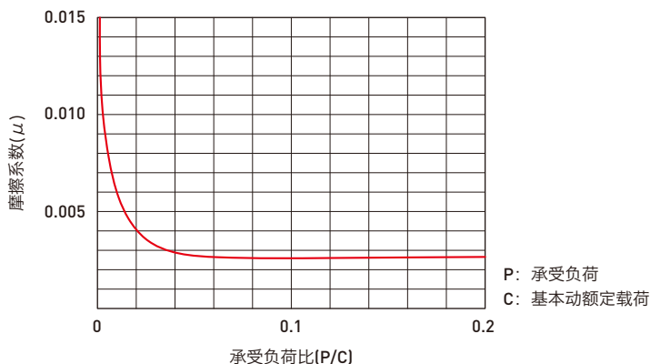
■ 承受负荷与摩擦系数关系图
