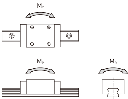
■ 各方向的力矩
