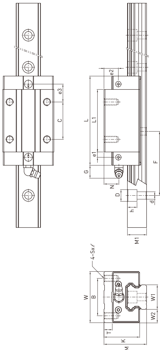
LMG...H / LH 型号尺寸表
